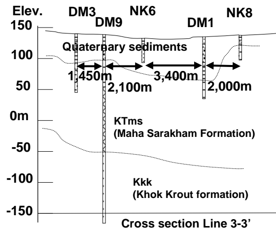
รูปที่ 6 รูปตัดตามแนว 3-3
